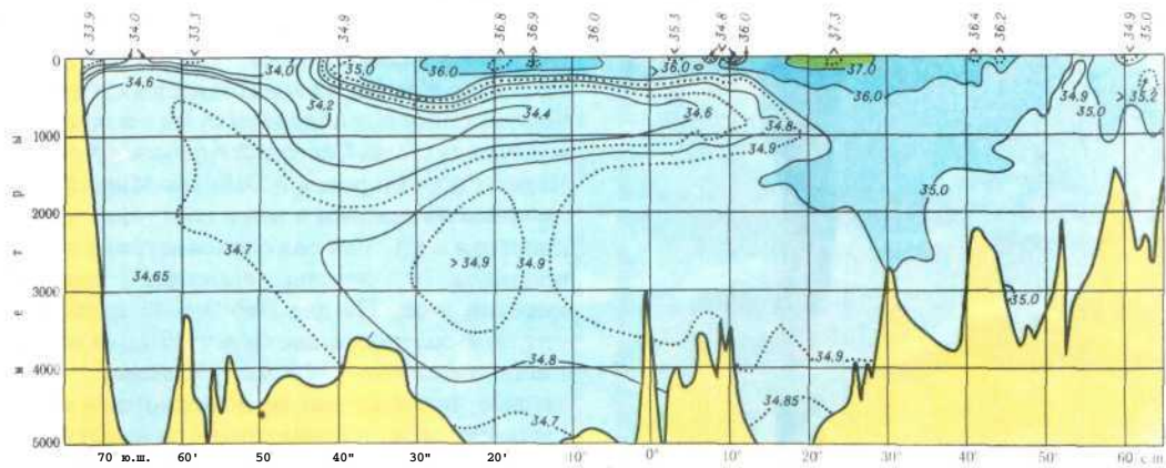
Вертикальный разрез солености через Атлантический океан
